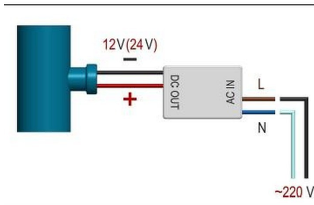
Schéma zapojenia osvetlenia: vývod kábla cez T-kus 75 × 50 × 75 mm, napájací zdroj 220 / 12 V
