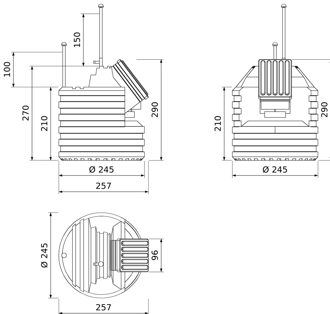
Záhradná pivnica 250 – tri pohľady, rozmery v centimetroch
