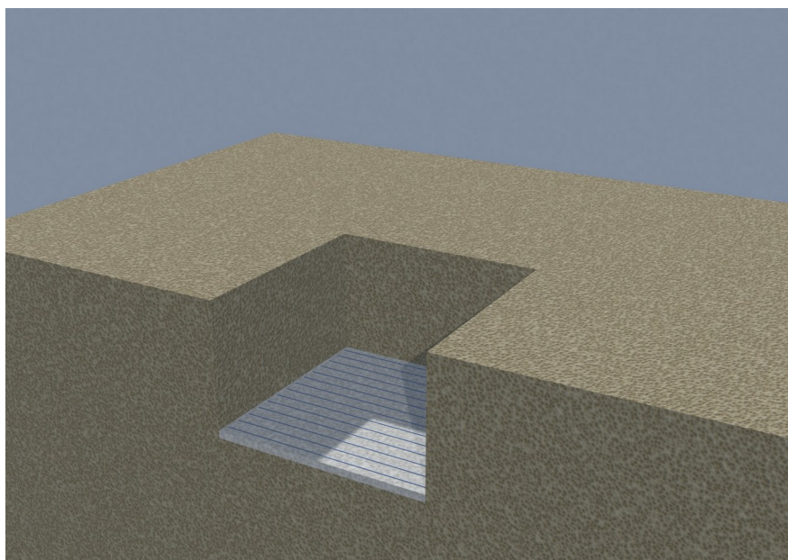
Krok 2. Vrstva suchého betónu 10 cm a prúty Ø12 mm s rozstupom 20 cm, od vstupu k zadnej časti
