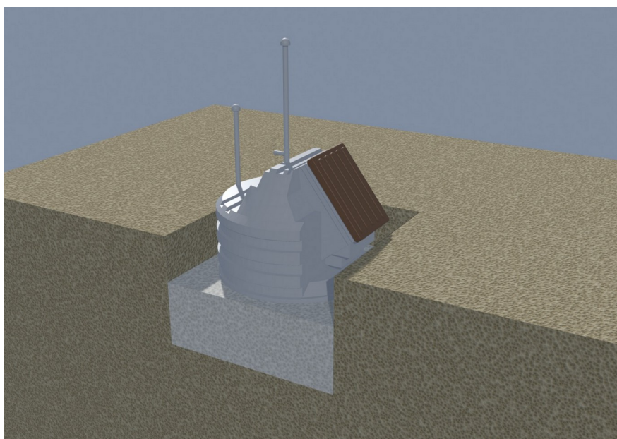
Krok 5. Obsyp suchým betónom do výšky 90 cm
