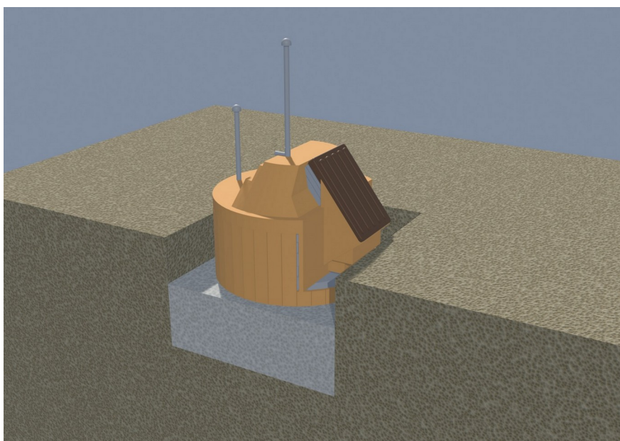
Krok 6. Zateplenie steny pásmi 20 cm, prednej časti a vstupu, XPS 5 cm
