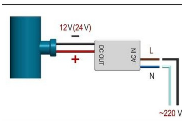
Schéma zapojenia osvetlenia: vývod kábla cez T-kus 100 × 50 × 100 mm, napájací zdroj 220 / 12 V
