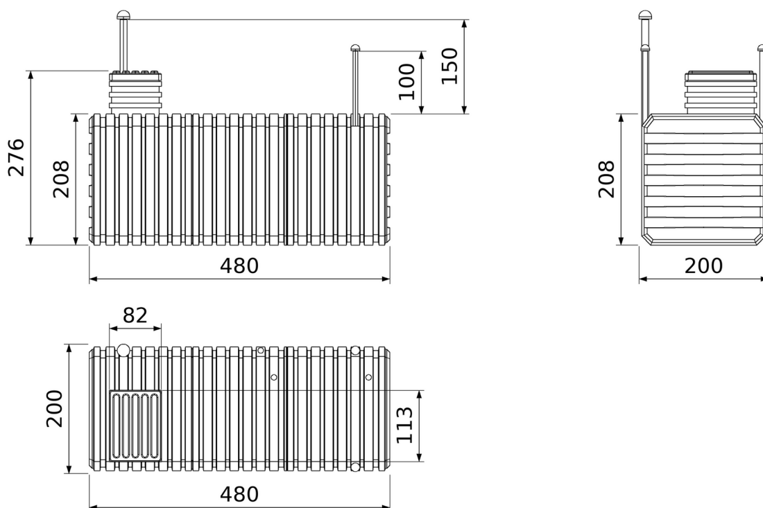
Záhradná pivnica 200 × 480 – tri pohľady, rozmery v centimetroch
