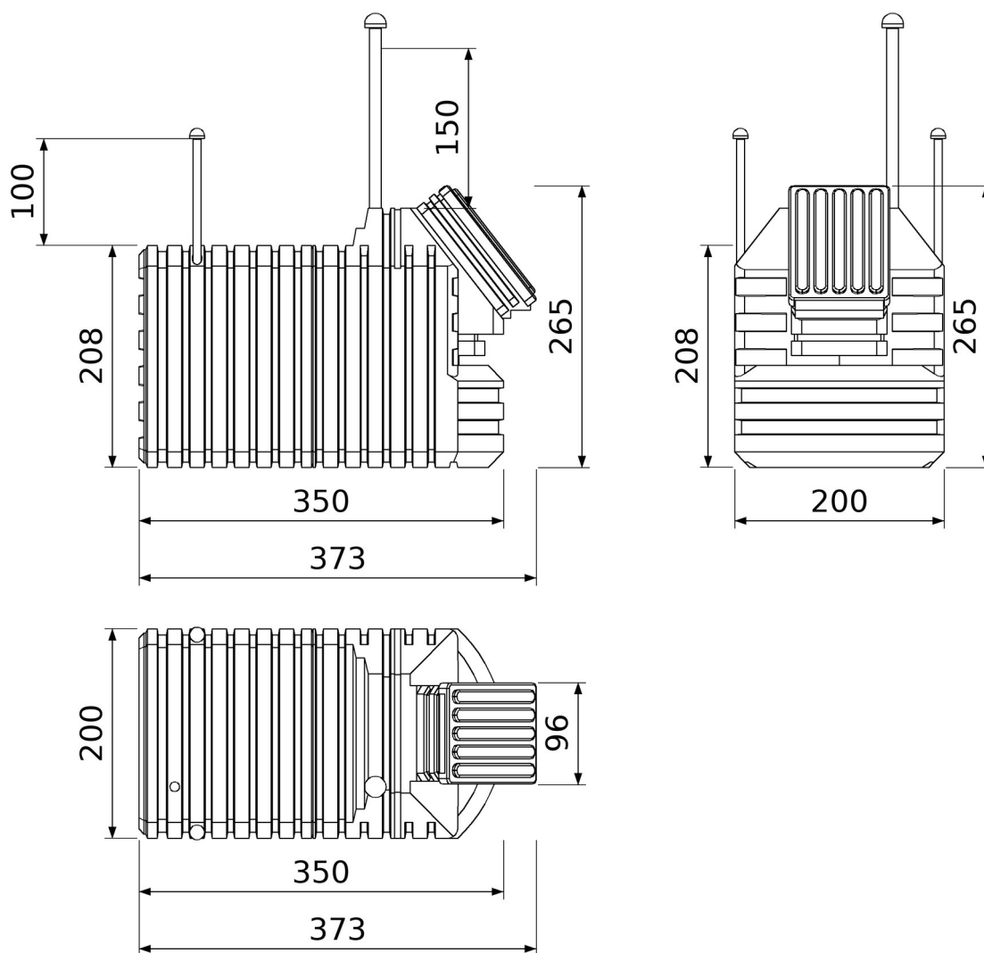
Vrtna klet 200 × 350 — tri projekcije, mere v centimetrih
