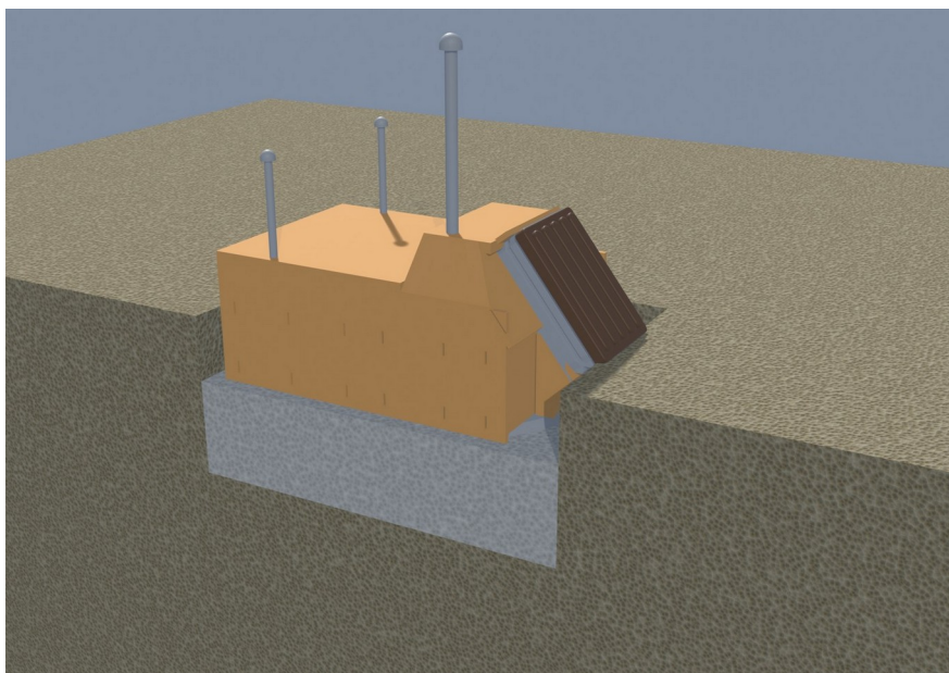
Korak 6. Toplotna izolacija stranic, čel, sprednjega dela in vhoda, XPS 5 cm
