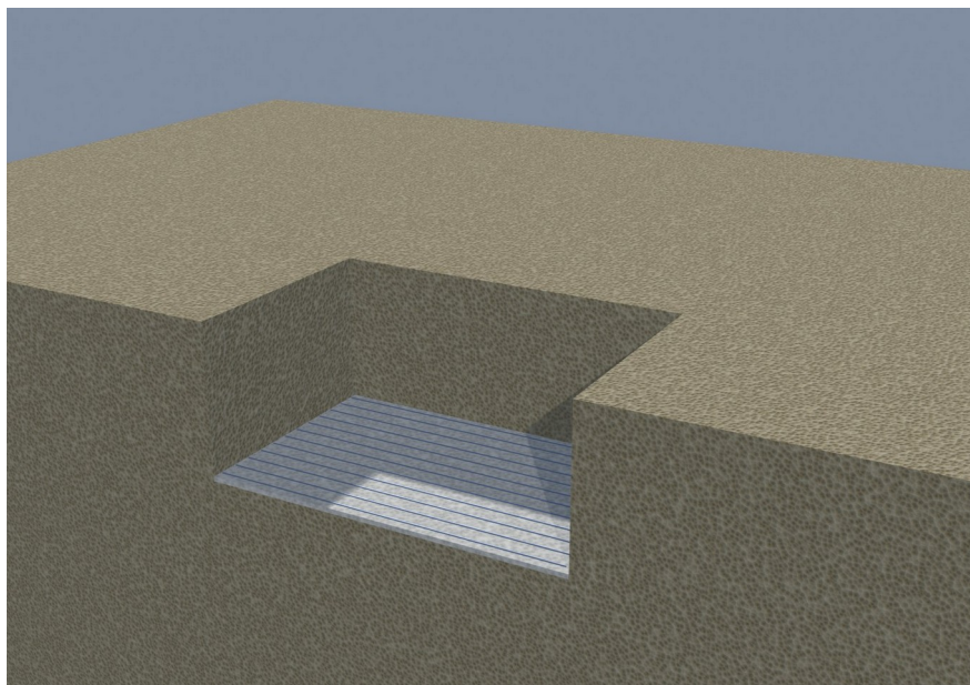
Korak 2. Sloj suhega betona 5 cm in vzdolžne palice Ø12 mm na razmiku 20 cm
