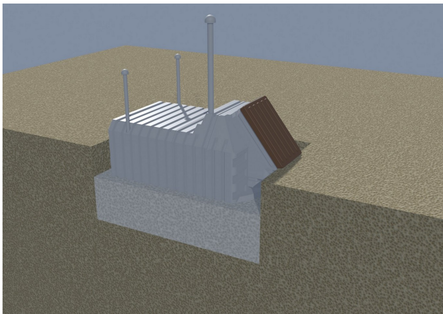
Korak 5. Obsip s suhim betonom do višine 88 cm
