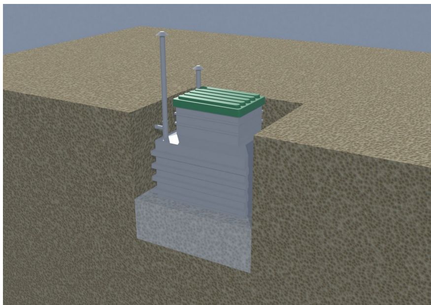
Korak 5. Obsip s suhim betonom do višine 58 cm
