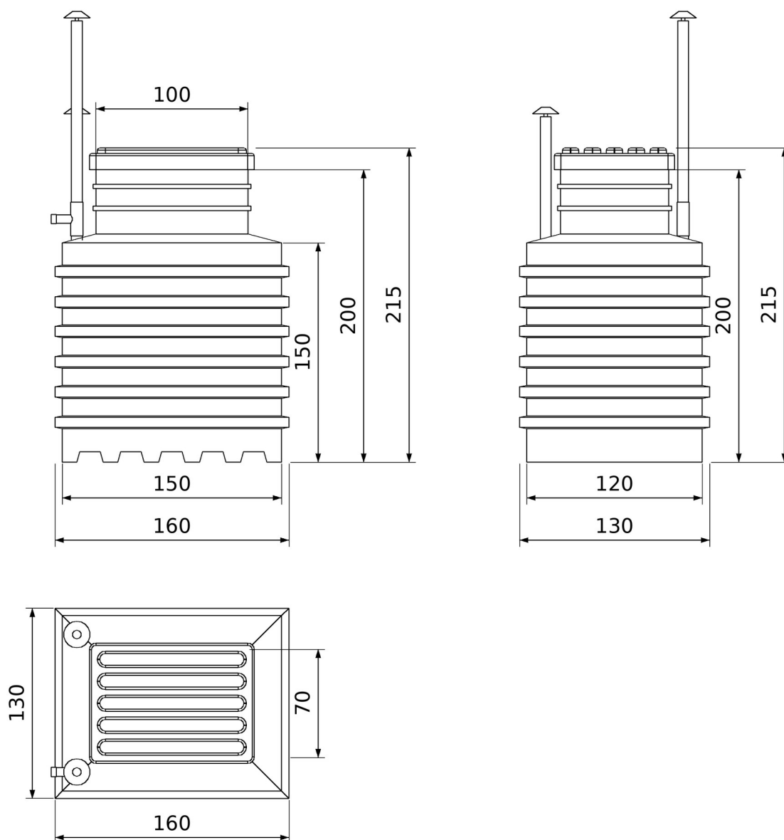
Vrtna klet 130 × 160 — tri projekcije, mere v centimetrih
