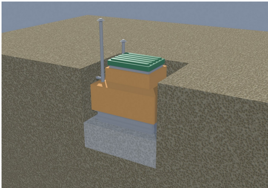
Korak 6. Toplotna izolacija vhoda, zgornjega dela in sten 60 cm, XPS 5 cm
