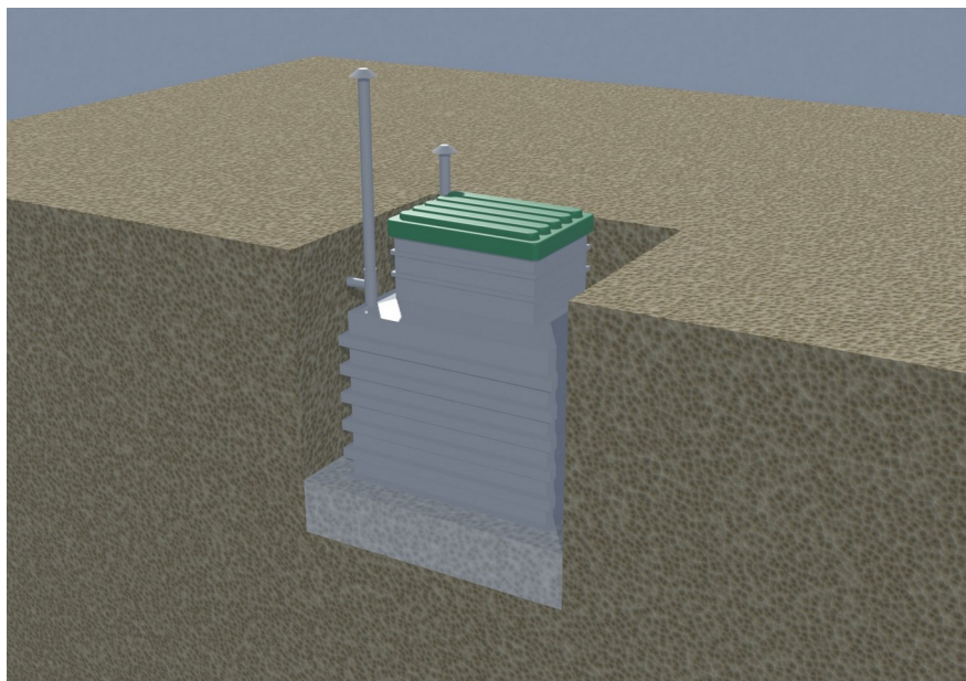
Korak 5. Prvi sloj suhega betona, 30 cm
