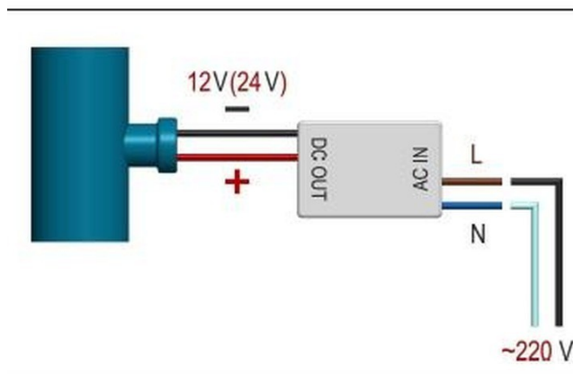
Koblingsskjema for belysningen: kabelutføring gjennom T-rør 100 × 50 × 100 mm, strømforsyning 220 / 12 V
