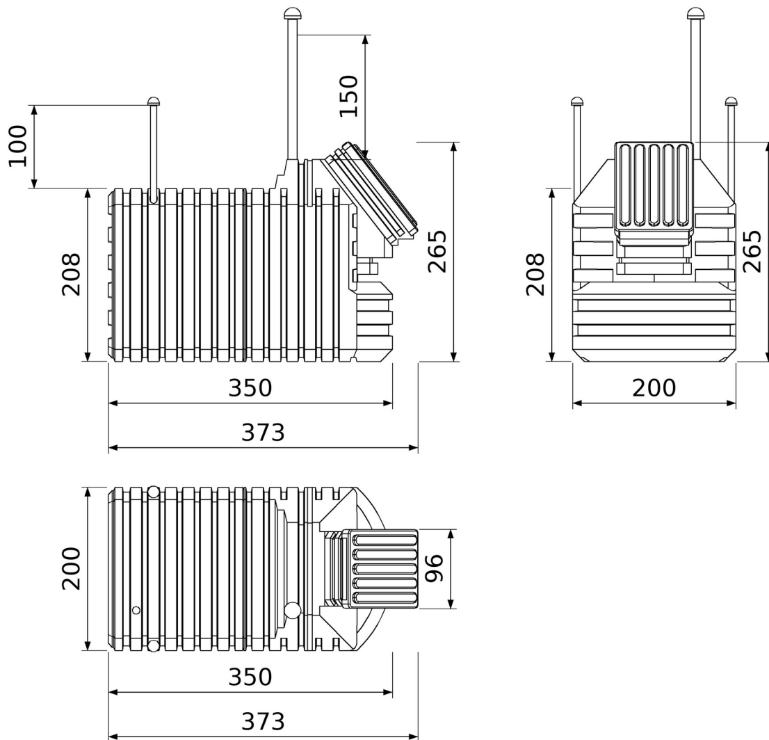
Jordkjeller 200 × 350 — tre projeksjoner, mål i centimeter
