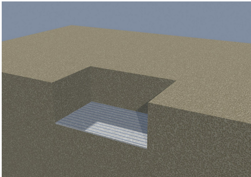
Trinn 2. Lag med tørrbetong 5 cm og langsgående jern Ø12 mm c/c 20 cm
