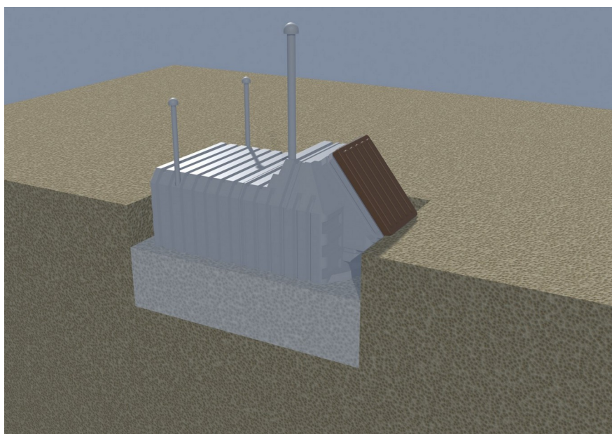
Trinn 5. Omfylling med tørrbetong opp til 88 cm
