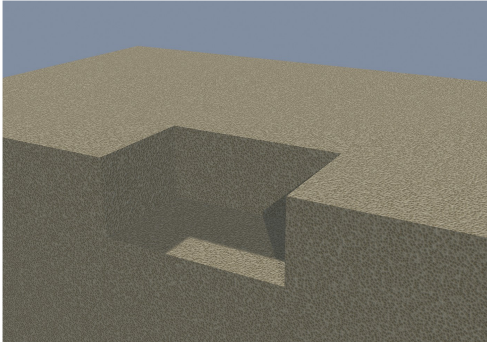
Trinn 1. Byggegrøp 385 × 240 cm, dybde 165 cm
