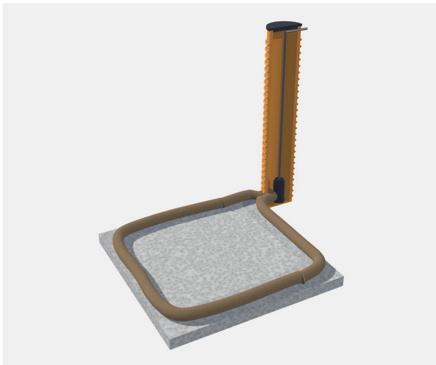
Skisse av dreneringssystemet: bunnplate, ringdrensrør, kum i snitt, pumpe og trykkledning
