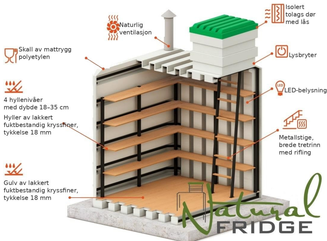
Kjelleren i snitt: hyller, stige, belysning og ventilasjon
