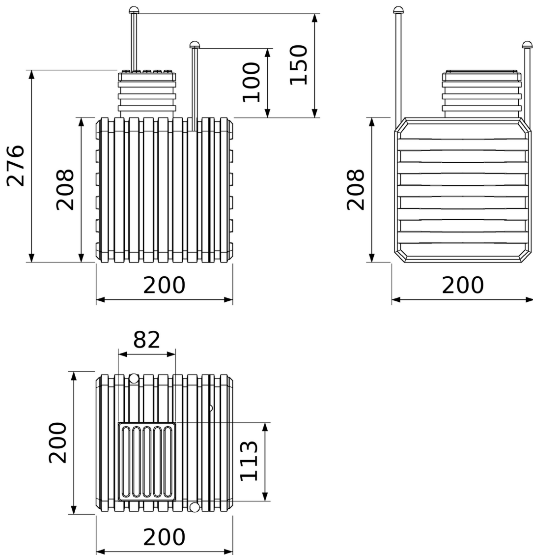
Jordkjeller 200 × 200 — tre projeksjoner, mål i centimeter
