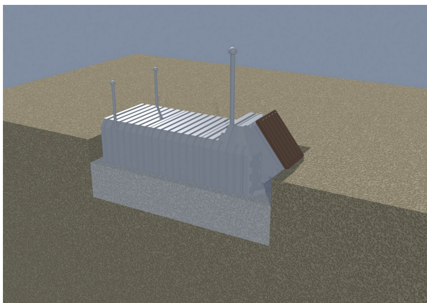
Stap 5. Omstorting met droogbeton tot 88 cm hoogte
