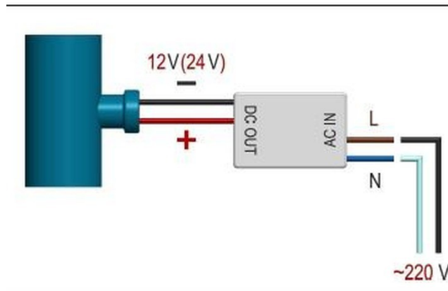
Aansluitschema verlichting: kabeldoorvoer via T-stuk 100 × 50 × 100 mm, voeding 220 / 12 V
