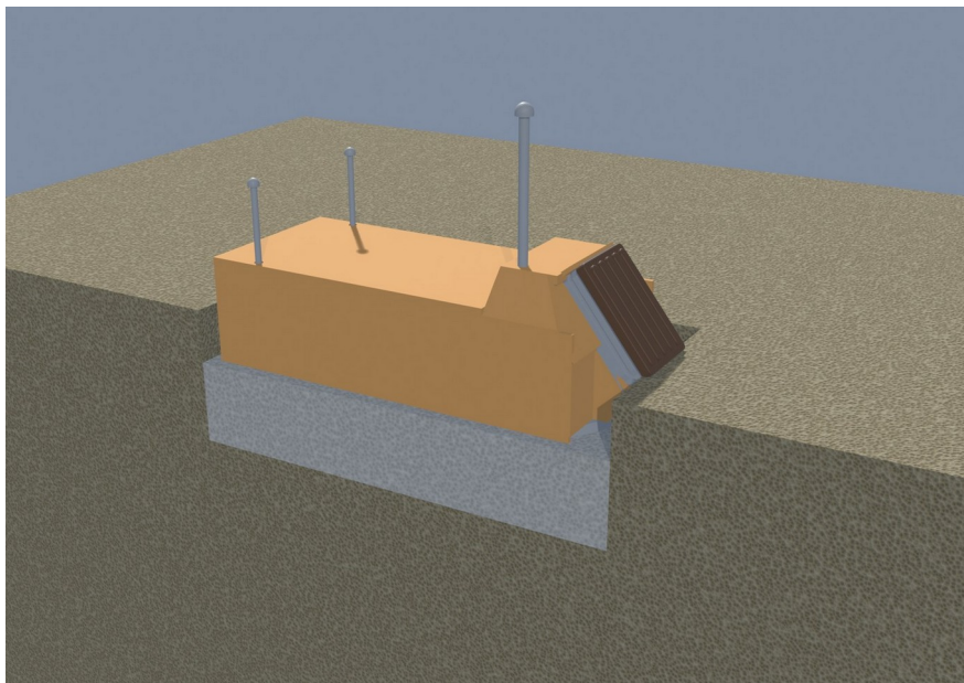
Stap 6. Isolatie zij- en kopwanden, voorzijde en ingang, XPS 5 cm
