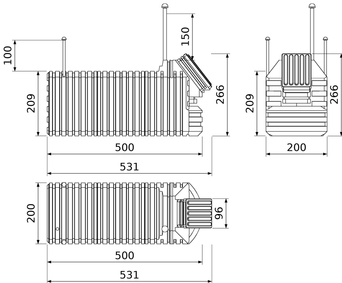
Tuinkelder 200 × 500 — drie aanzichten, maten in centimeters
