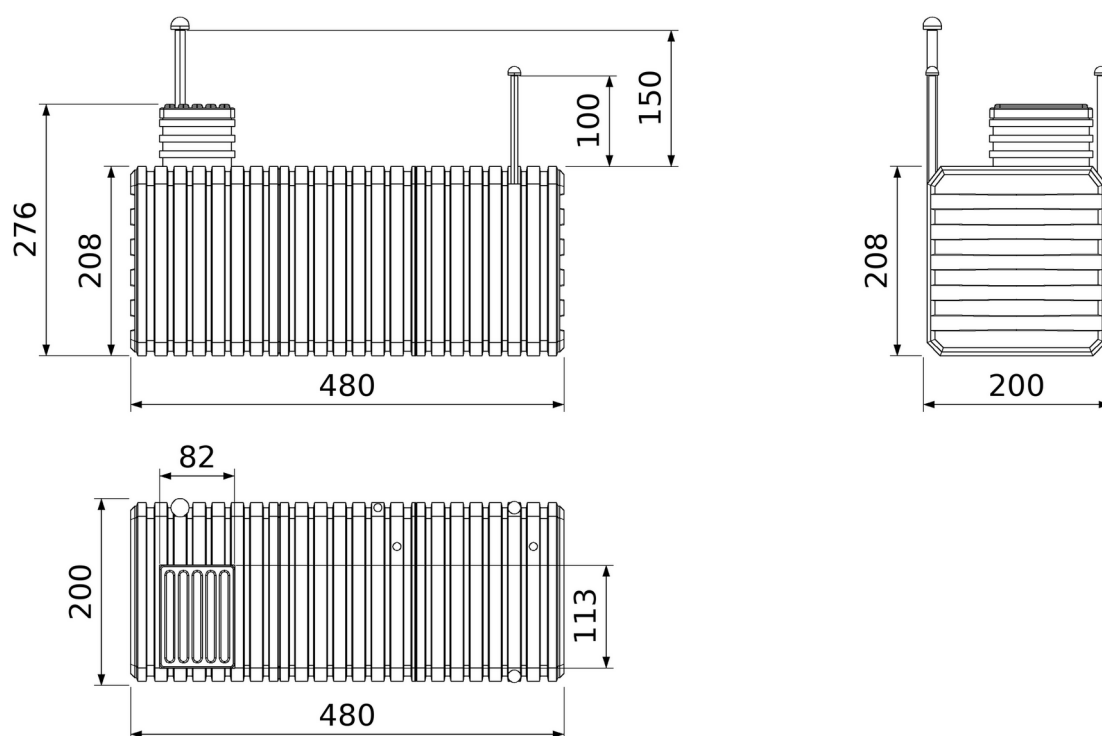
Tuinkelder 200 × 480 — drie aanzichten, maten in centimeters
