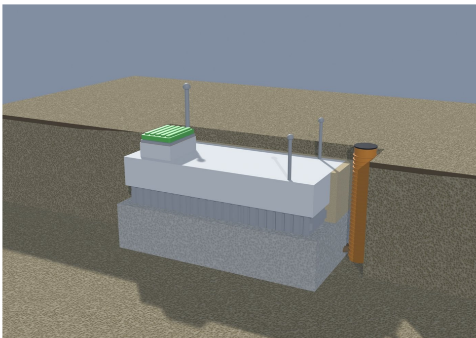
Stap 10. Aanvullen met zand, in doorsnede
