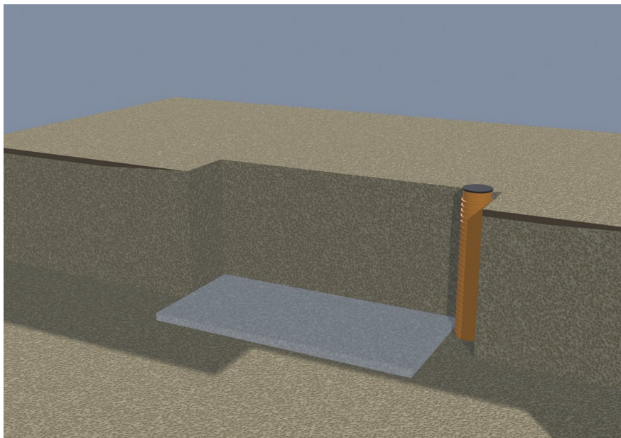
Stap 3. Drainageput in de uitgraving
