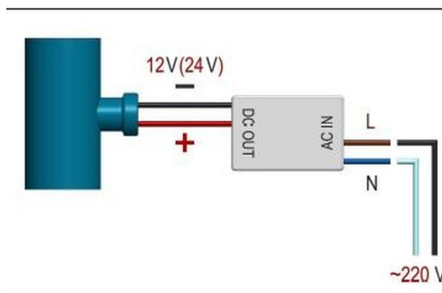
Aansluitschema verlichting: kabeldoorvoer via T-stuk 100 × 50 × 100 mm, voeding 220 / 12 V
