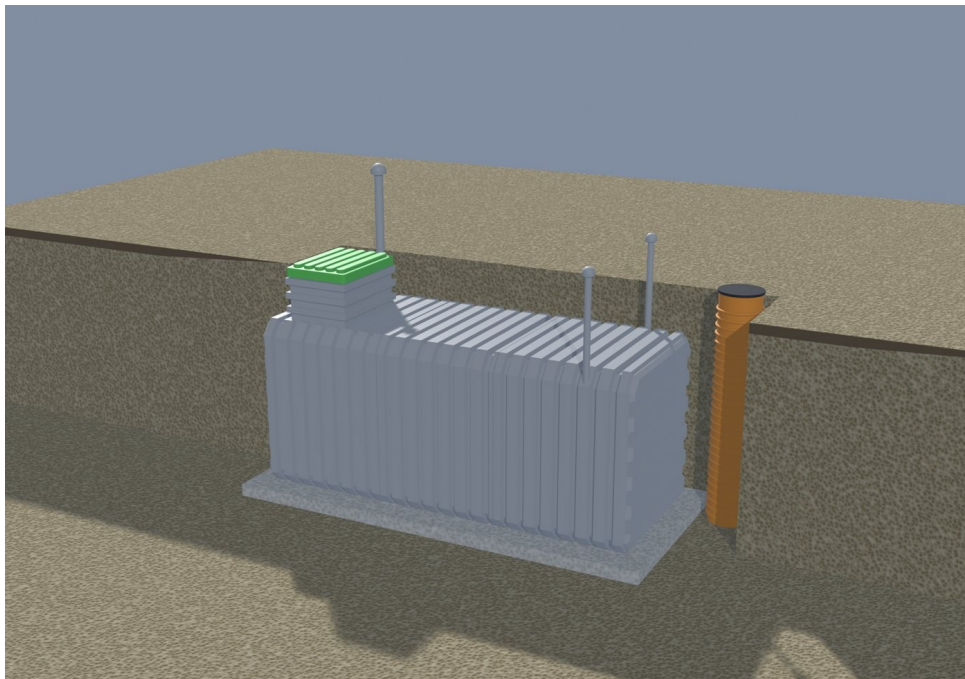
Stap 4. Behuizing op de bodemplaat geplaatst
