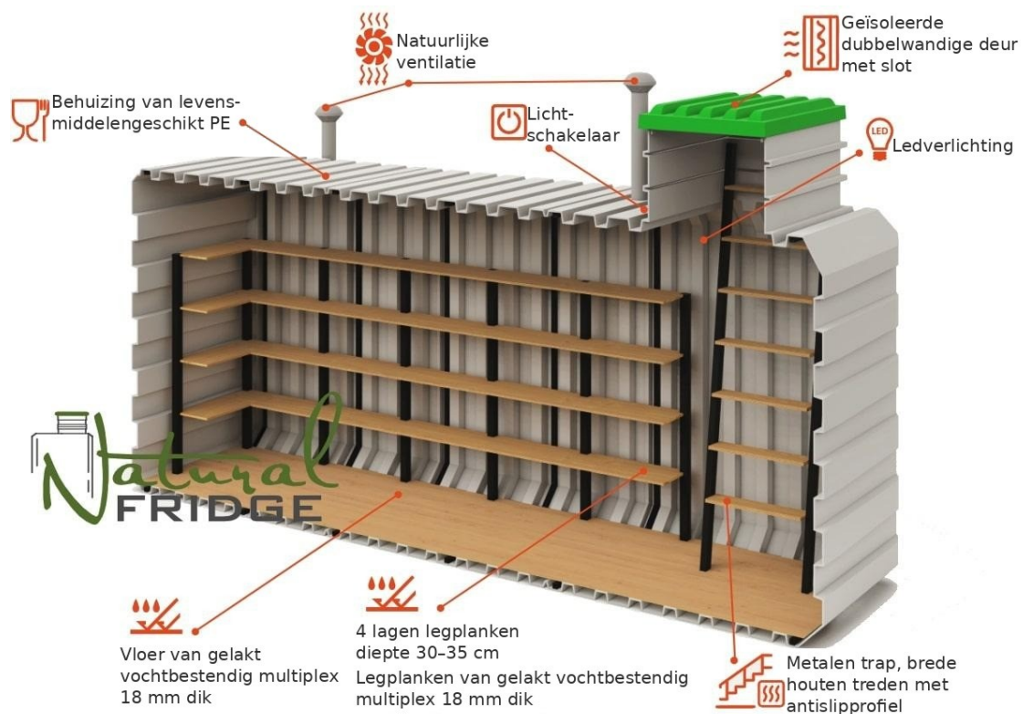
Doorsnede van de kelder: legplanken, trap, verlichting en ventilatie
