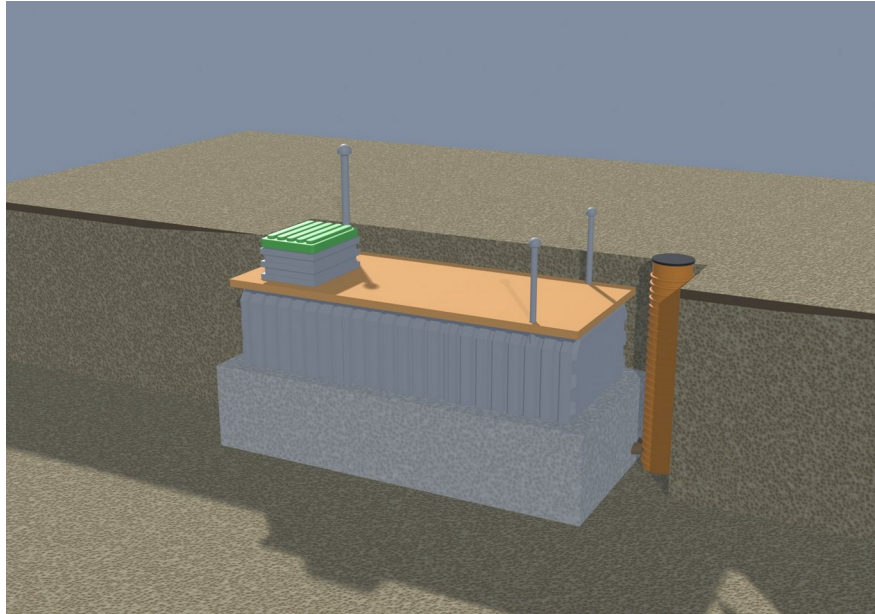
Stap 8. Isolatie bovenzvlak, XPS 10 cm
