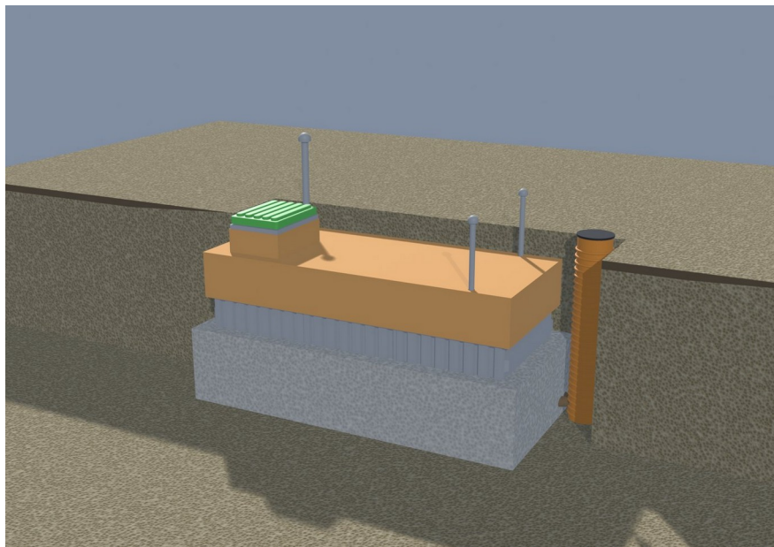
Stap 8. Isolatie zij- en kopwanden en ingang, XPS 5 cm
