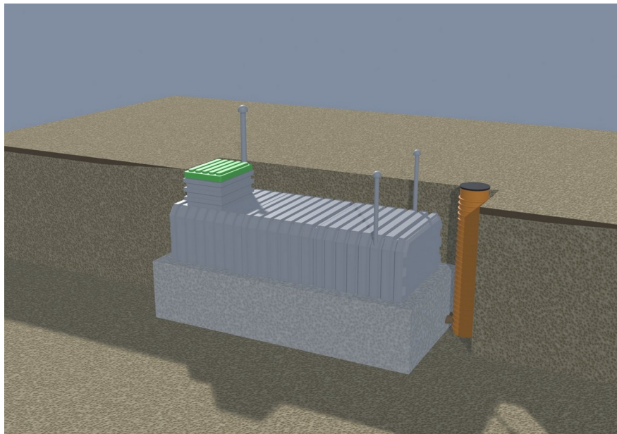
Stap 7. Omstorting met droogbeton tot 1 m hoogte
