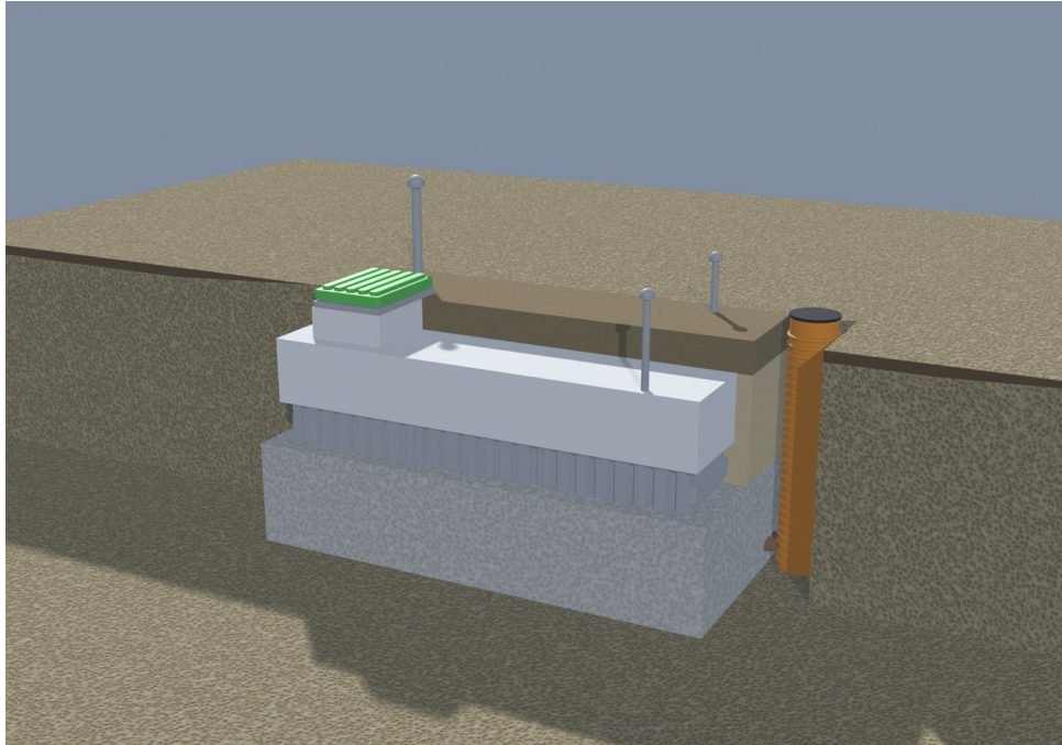
Stap 11. Aanvullen met grond, in doorsnede
