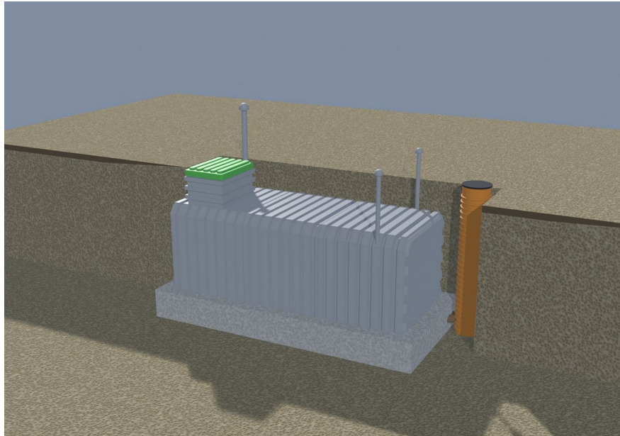
Stap 7. Eerste laag droogbeton, 40 cm
