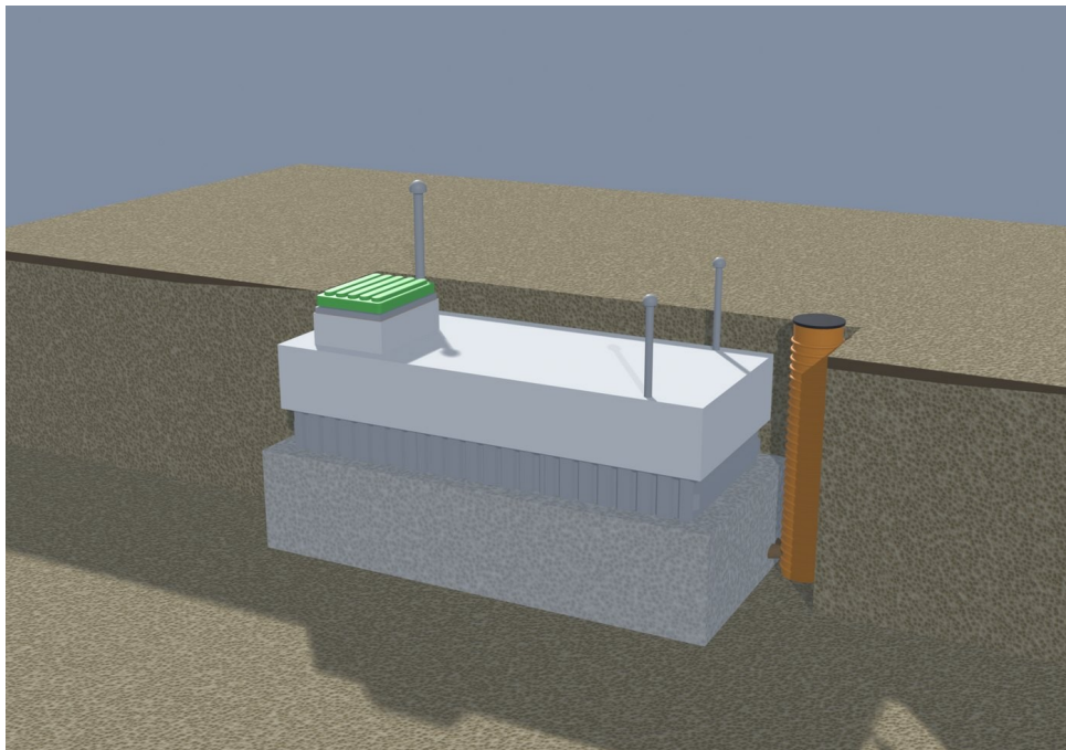
Stap 9. Isolatie afgedekt met geotextiel
