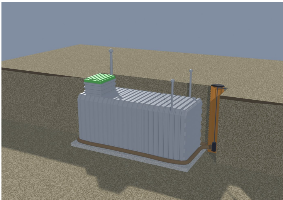
Stap 5. Ringdrainagebuis, pomp en persleiding
