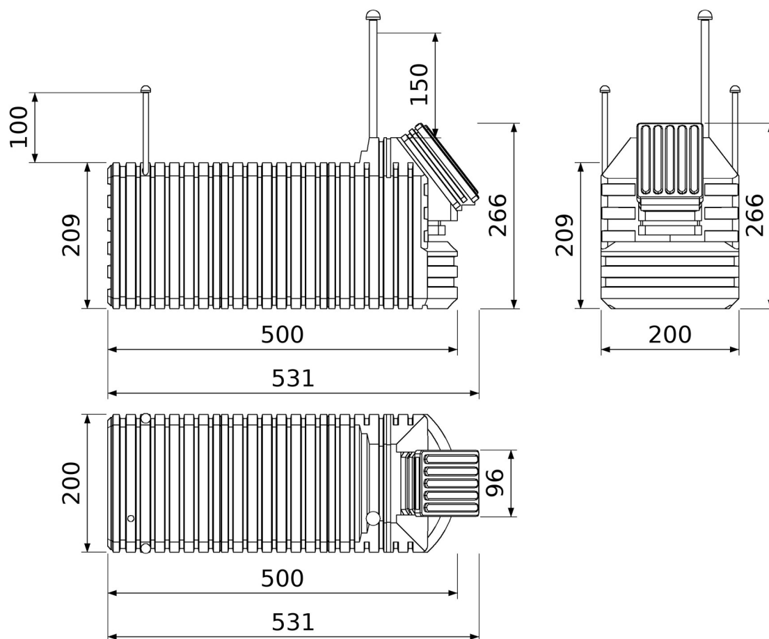
Sodo rūsys 200 × 500 – trys projekcijos, matmenys centimetrais
