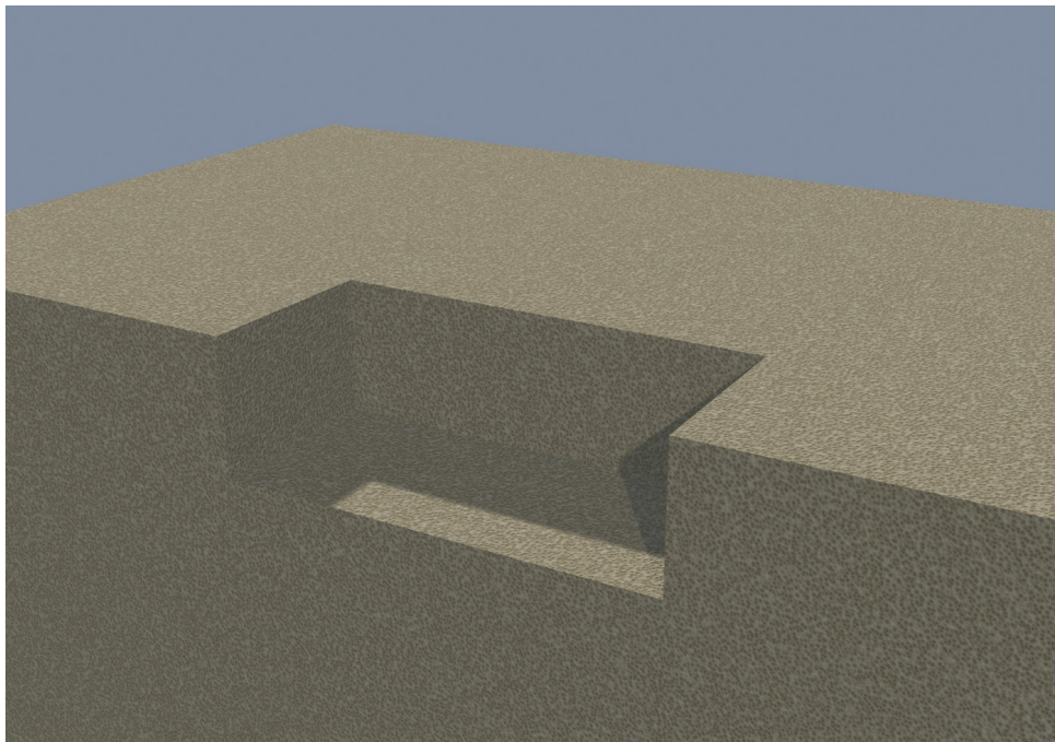
1 etapas. Duobė 540 × 240 cm, 170 cm gylis
