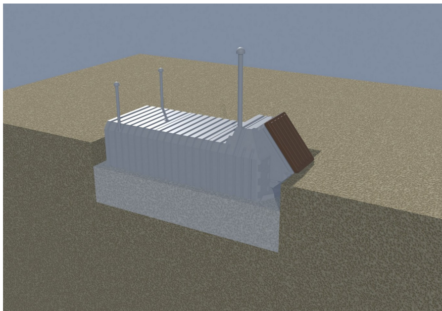
5 etapas. Apipylimas sausu betonu iki 88 cm aukščio
