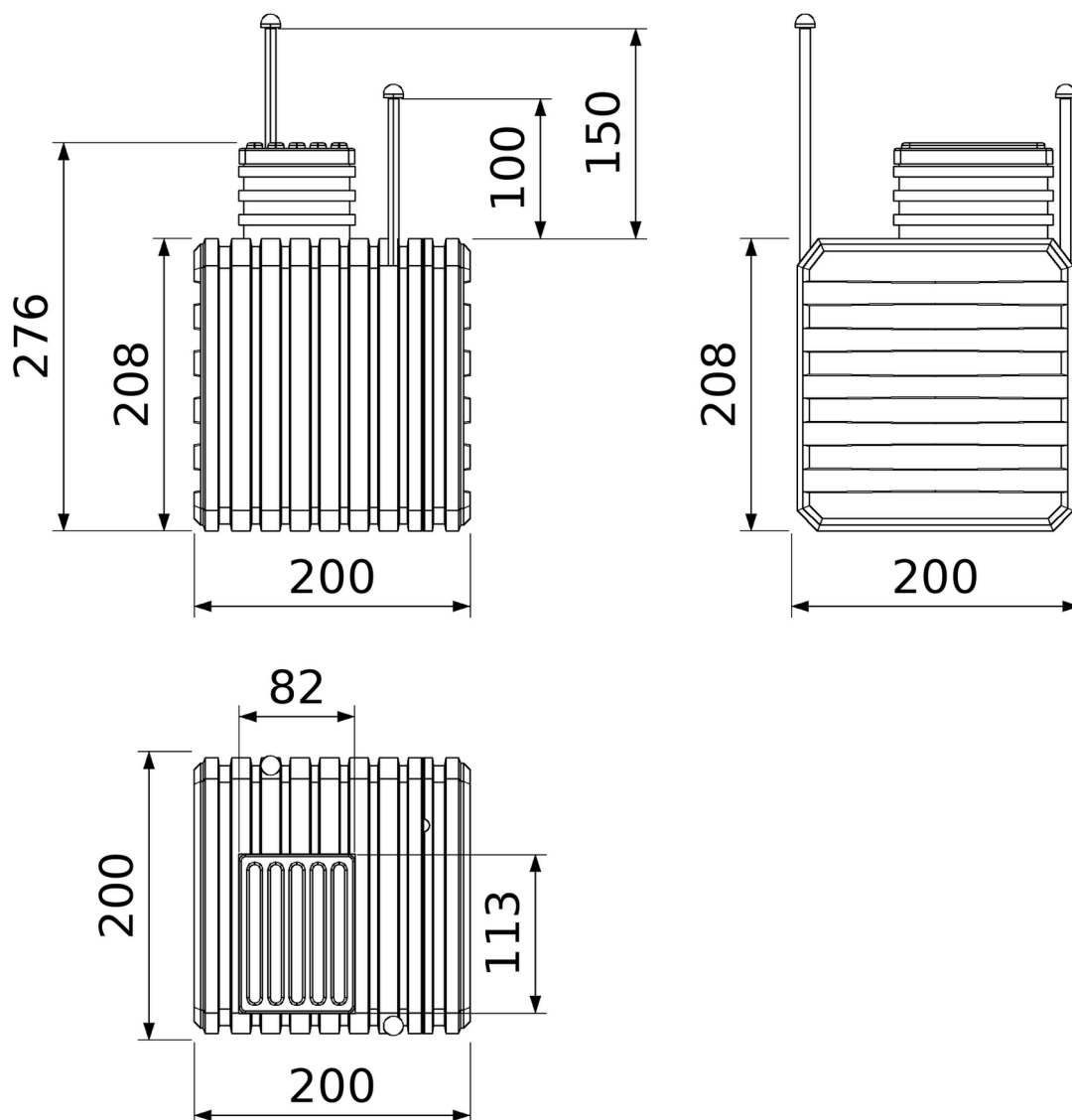
Sodo rūsys 200 × 200 – trys projekcijos, matmenys centimetrais
