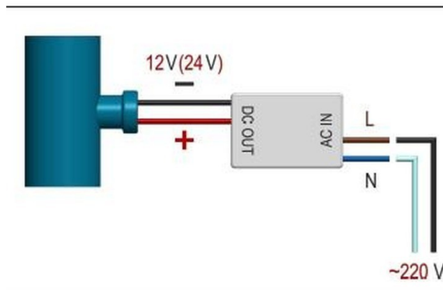
Schéma de raccordement de l'éclairage : sortie du câble par le té 75 × 50 × 75 mm, bloc d'alimentation 220 / 12 V
