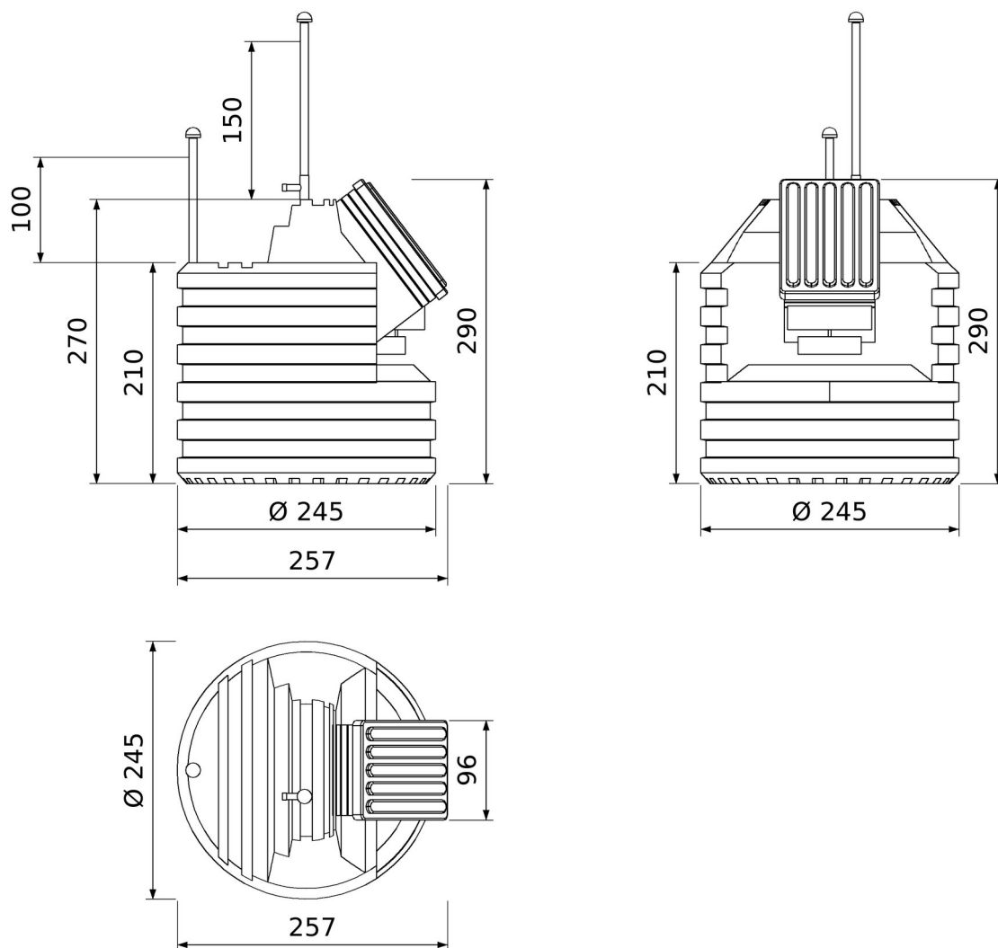
Cave de jardin 250 — trois vues, cotes en centimètres
