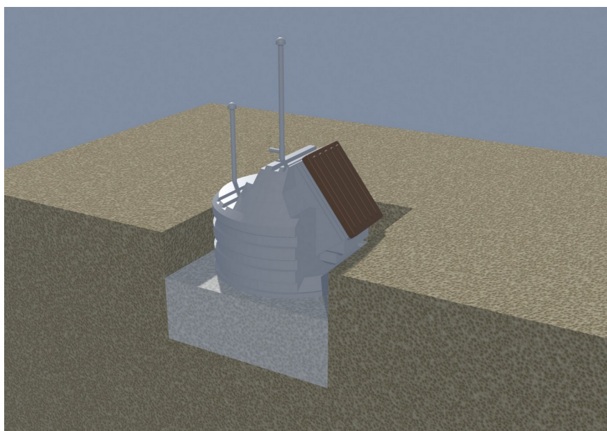
Étape 5. Enrobage en béton sec jusqu'à 90 cm de hauteur
