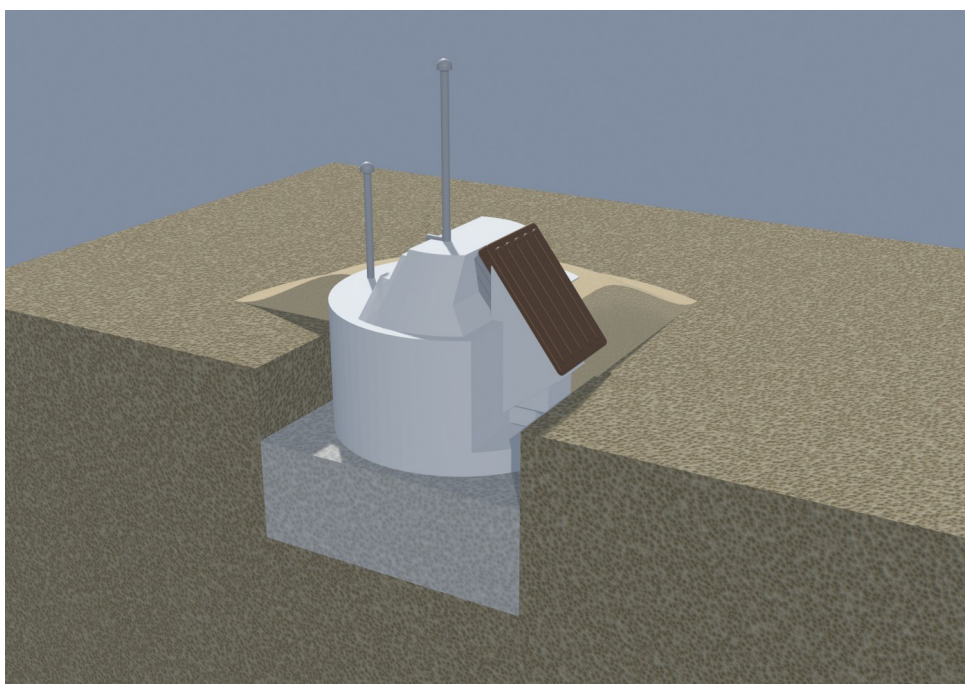
Étape 8. Remblaiement au sable, vue en coupe
