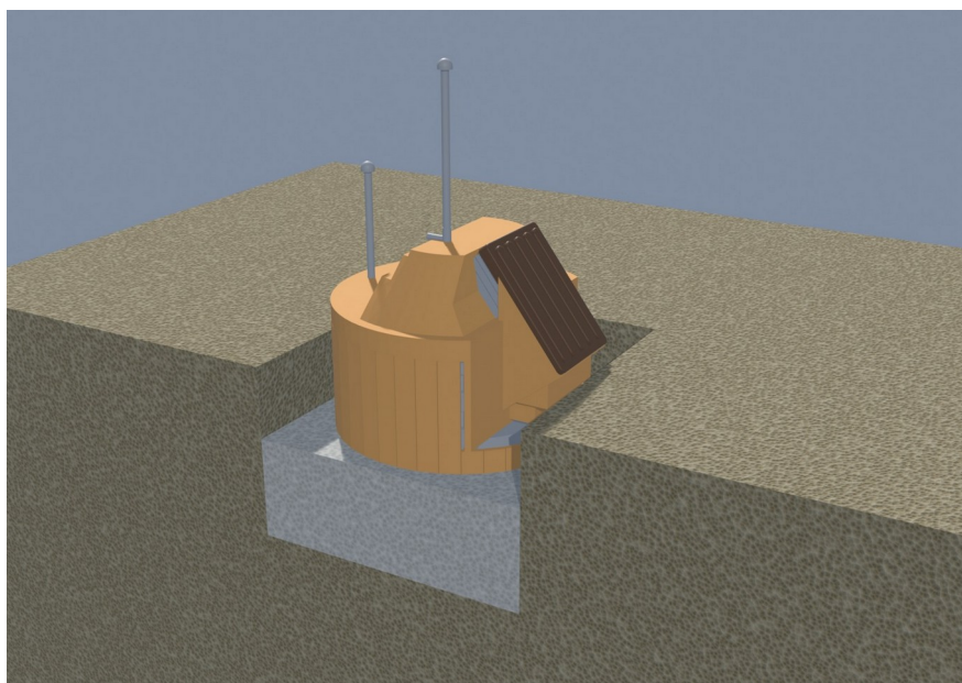
Étape 6. Isolation de la paroi en bandes de 20 cm, de la partie avant et de l'entrée, XPS 5 cm
