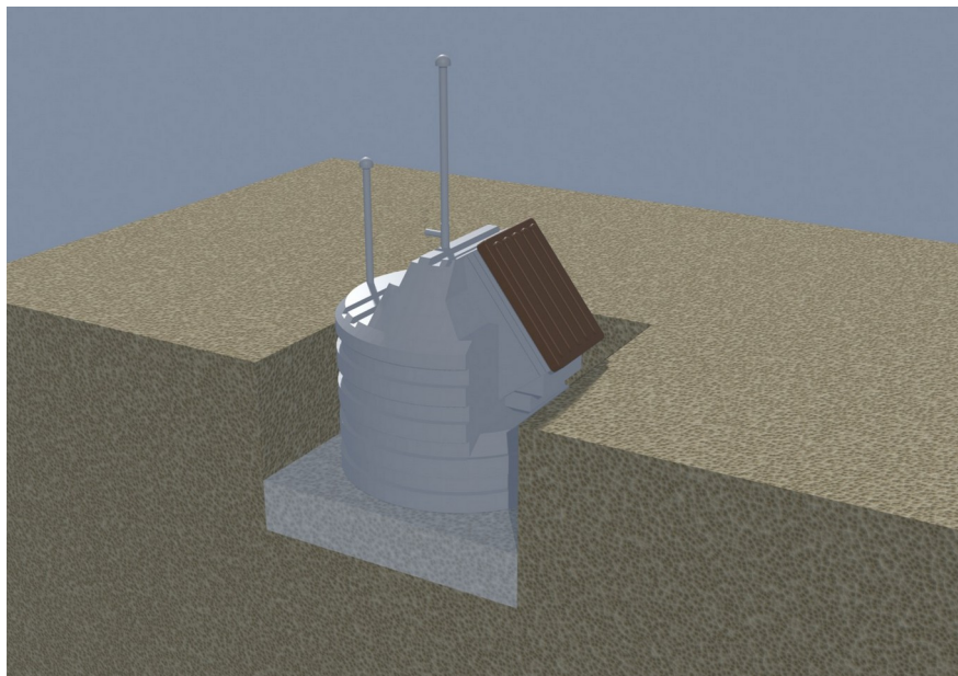
Étape 5. Première couche de béton sec, 40 cm
