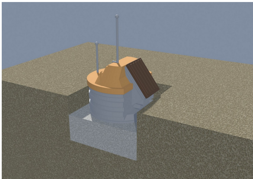
Étape 6. Isolation de la face supérieure et de la partie surélevée, XPS 10 cm
