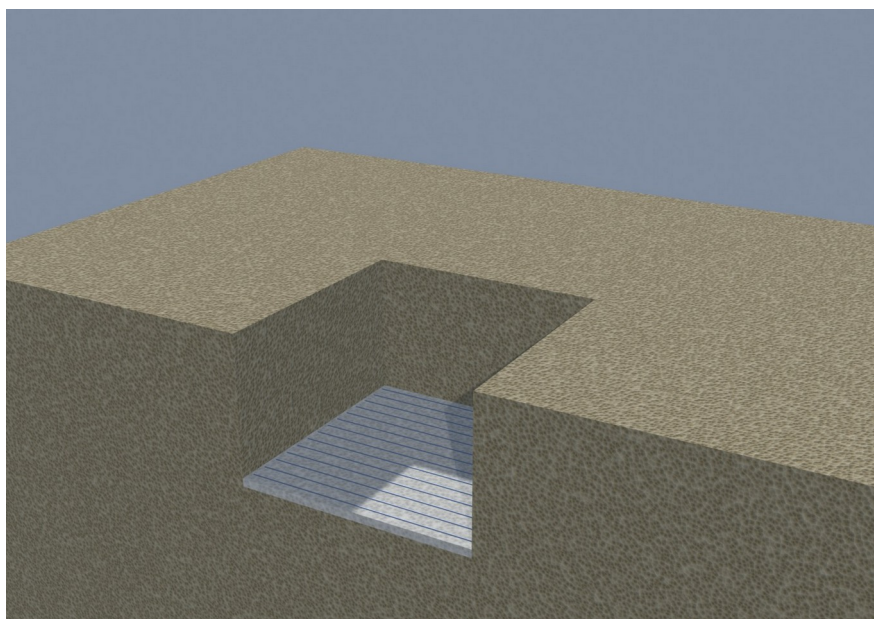
Étape 2. Couche de béton sec de 10 cm et barres Ø12 mm espacées de 20 cm, de l'entrée vers l'arrière
