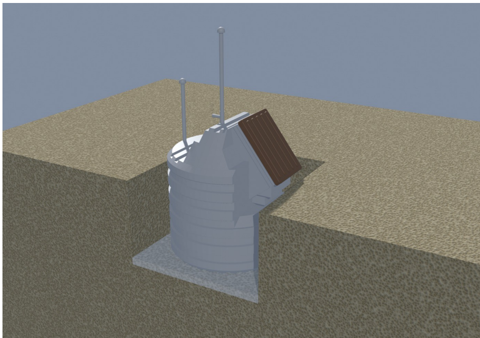
Étape 3. Coque posée sur la dalle
