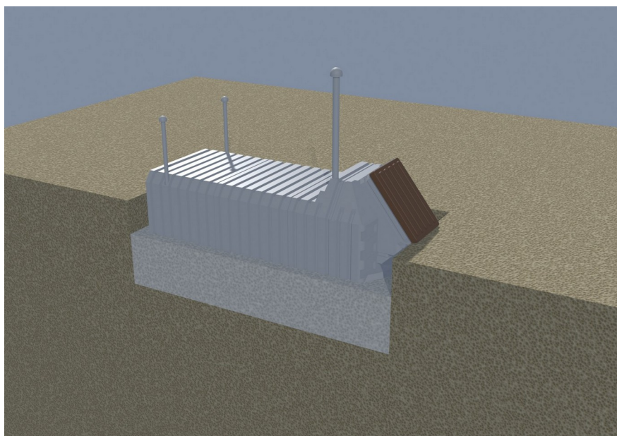
Étape 5. Enrobage en béton sec jusqu'à 88 cm de hauteur
