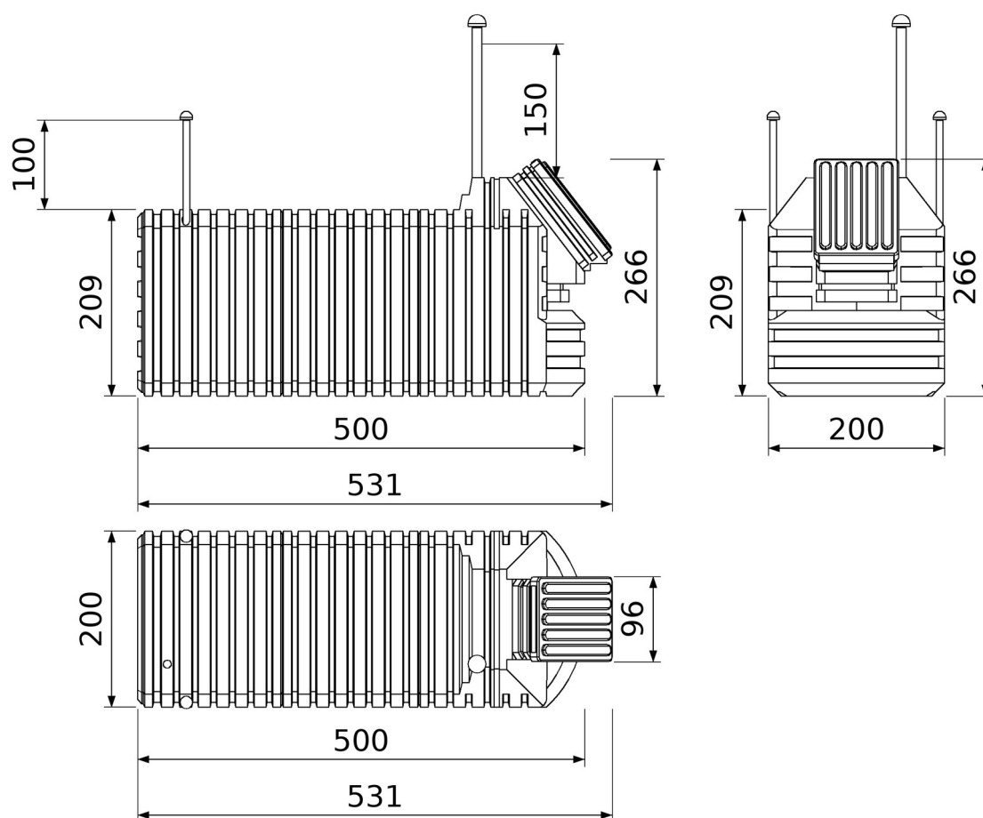
Cave de jardin 200 × 500 — trois vues, cotes en centimètres
