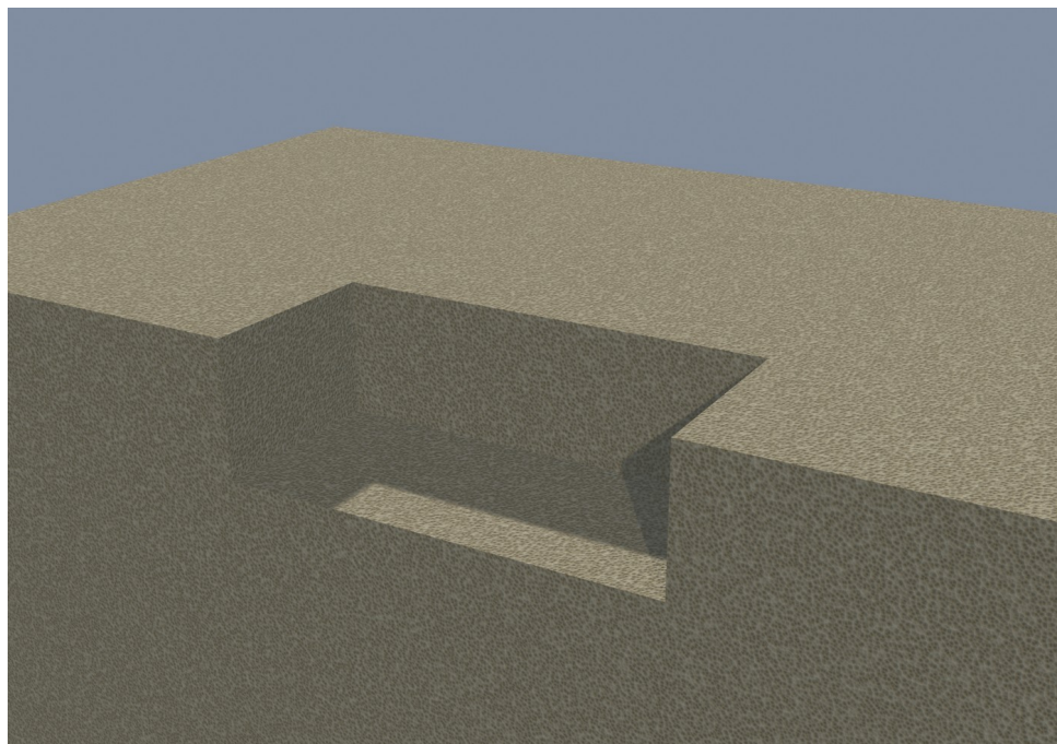
Étape 1. Fouille de 540 × 240 cm, profondeur 170 cm
