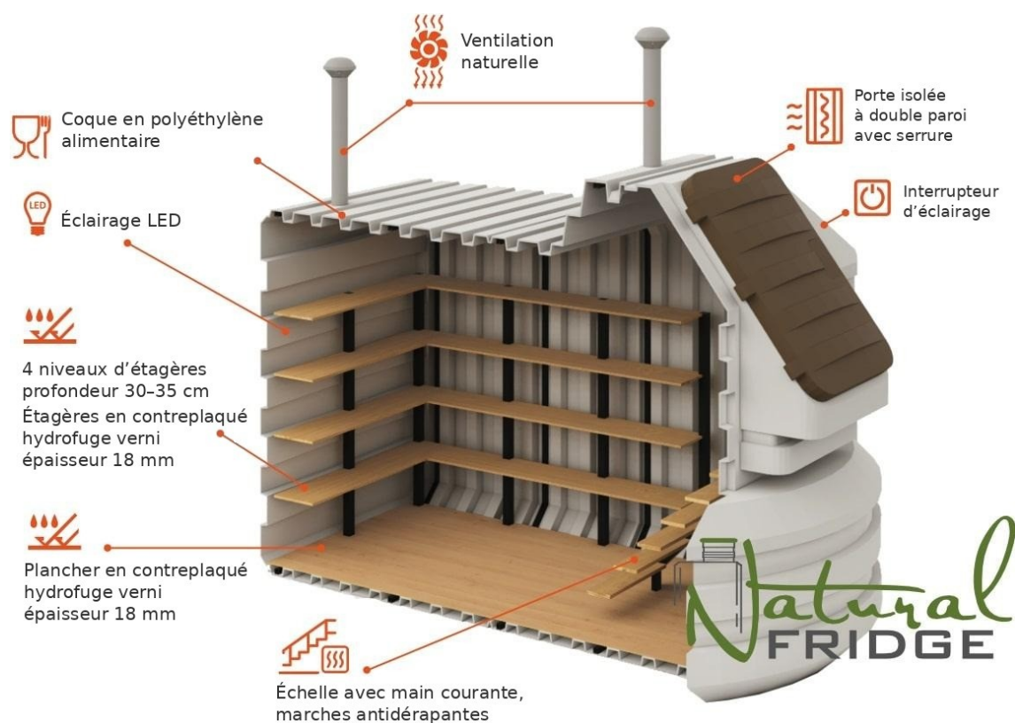
Cave en coupe : étagères, échelle, éclairage et ventilation
