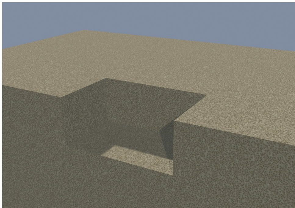
Étape 1. Fouille de 385 × 240 cm, profondeur 165 cm
