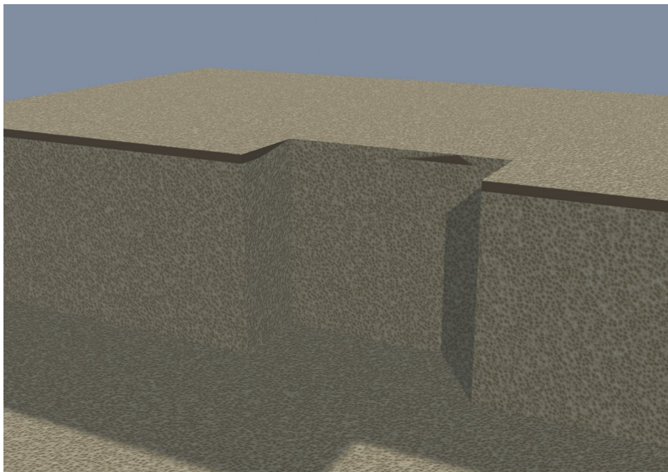
Étape 1. Fouille de 240 × 240 cm, profondeur 268 cm, et fosse du puisard
