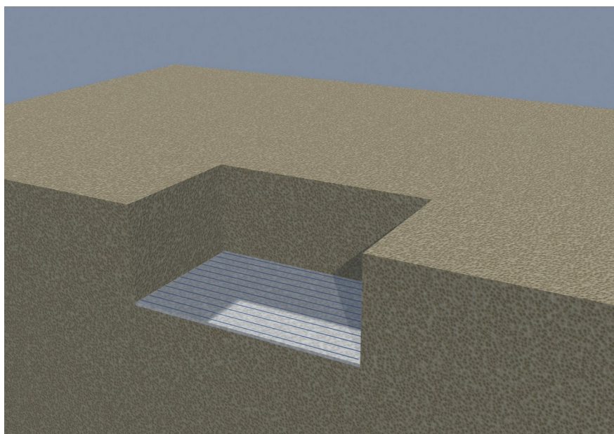
Trin 2. Lag tørbeton 5 cm og langsgående jern Ø12 mm med afstand 20 cm
