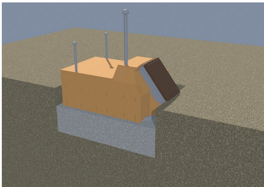
Trin 6. Isolering af sider, gavle, forende og indgang, XPS 5 cm
