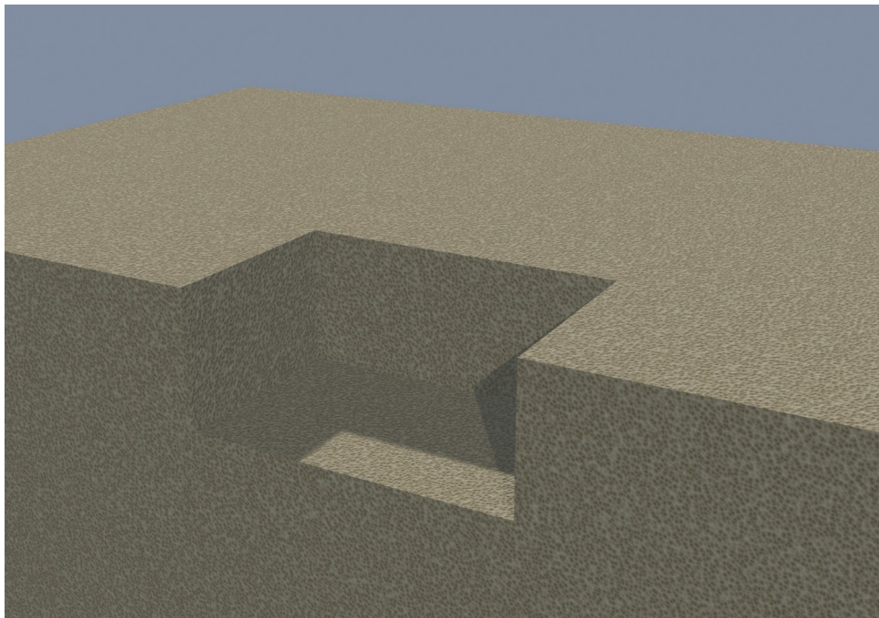
Trin 1. Byggegrube 385 × 240 cm, dybde 165 cm
