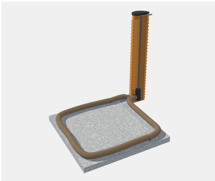
Skitse af drænsystemet: bundplade, omfangsdræn, brønd i snit, pumpe og trykledning
