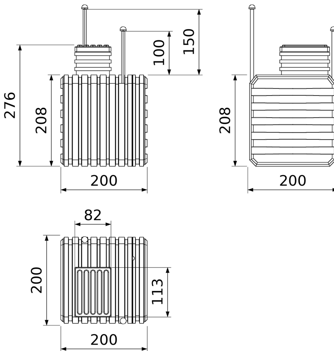
Havekælder 200 × 200 – tre visninger, mål i centimeter
